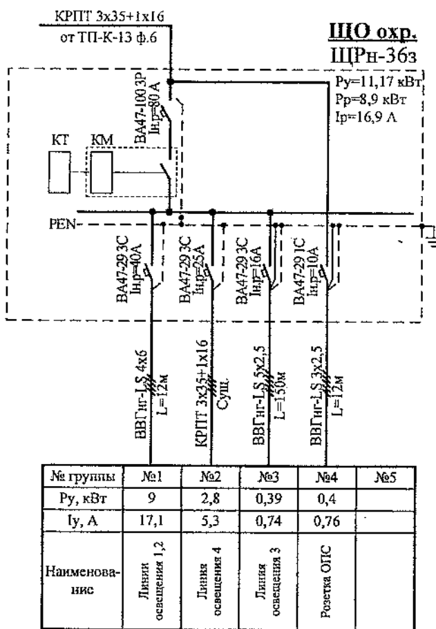
Рис. 1. Однолинейная схема ЩО охр.
